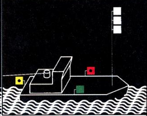
Každý z remorkerů v čele vlečné sestavy s více rem.
