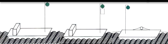
Remorkér v čele vlečné sestavy
