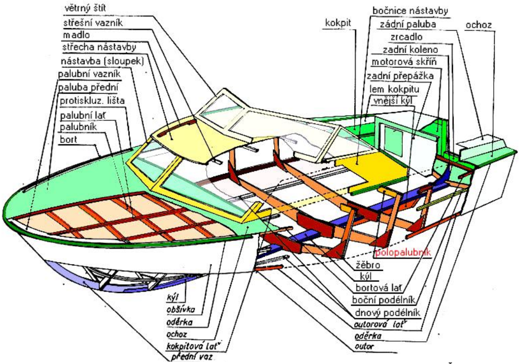
Konstrukce otevřené dřevěné motorové lodi
