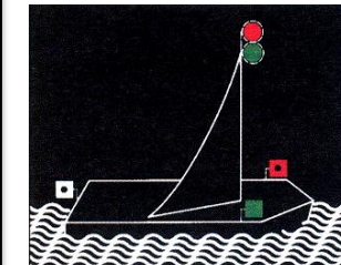
Plachetnice není malým plavidlem
