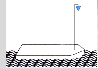
Plavidlo převážející nebezp. látky, dle počtu znaků: 10 / 50 / 100 m
